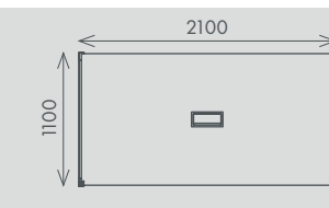
Mesa Reunião 8 pessoas (caixa elétrica opcional)
