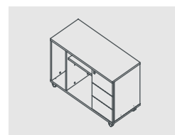
Armário Individual 1000 x 450 x 560
