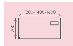
Mesa Linear (caixa elétrica opcional)
