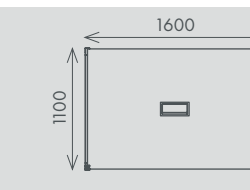
Mesa Reunião 6 pessoas (caixa elétrica opcional)
